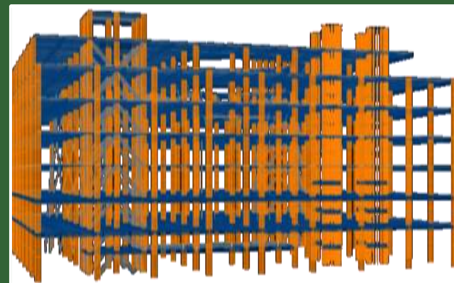
傳統梁柱鋼構系統
