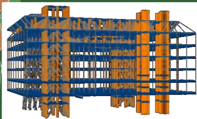
高圖鋼棒懸吊系統
